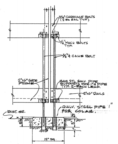
CANE BOLT DETAIL N.T.S. (12) C-11
